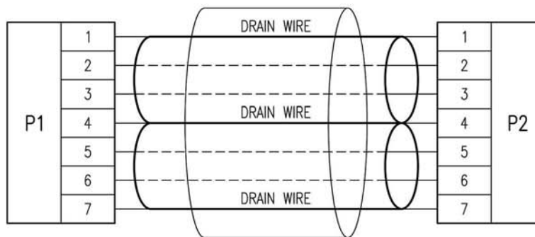
WIRING TABLE
